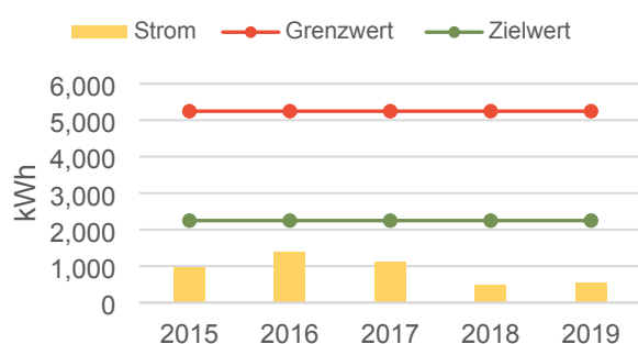
Verbrauchsentwicklung Strom
