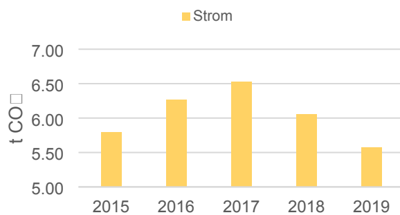
Entwicklung CO 2 -Emissionen Strom
